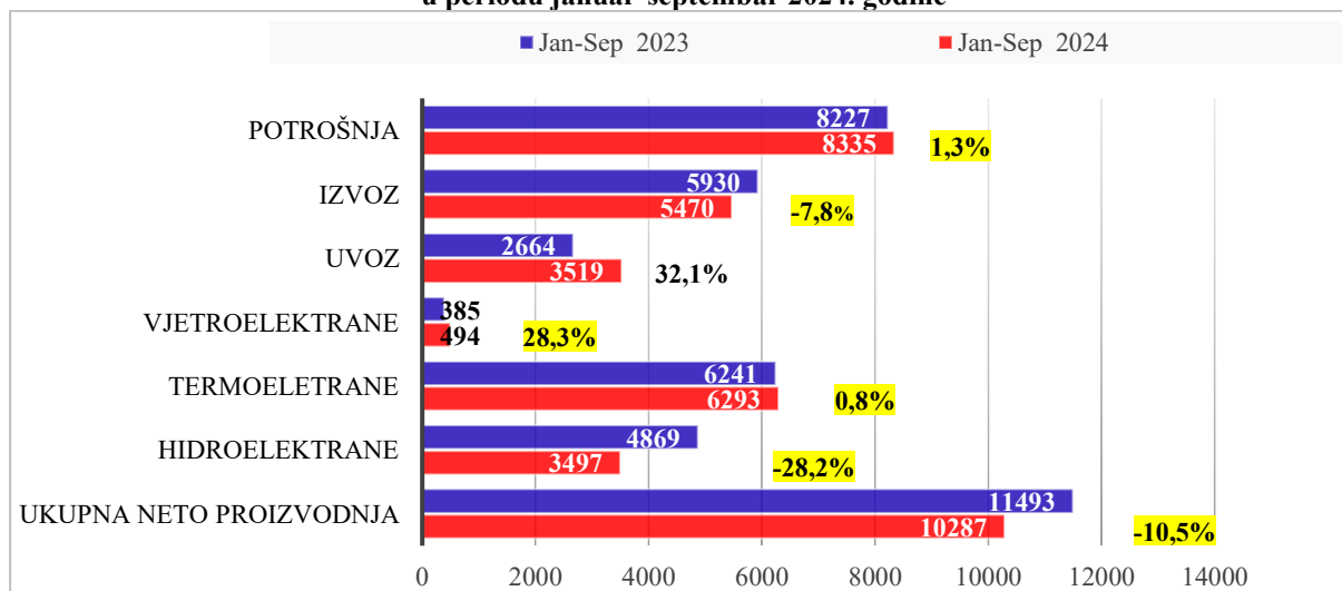
Grafikon 7: Pregled kretanja u sektoru za proizvodnju električne energije u periodu januar-septembar 2024. godine
