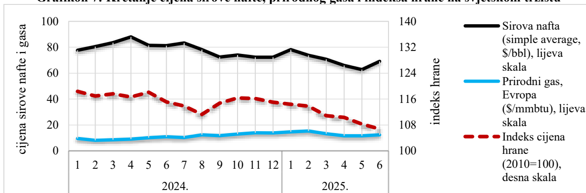
Grafikon 7: Kretanje cijena sirove nafte, prirodnog gasa i indeksa hrane na svjetskom tržištu
